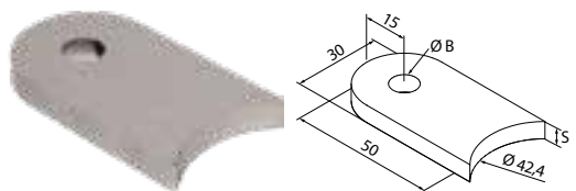
attacco da saldare
