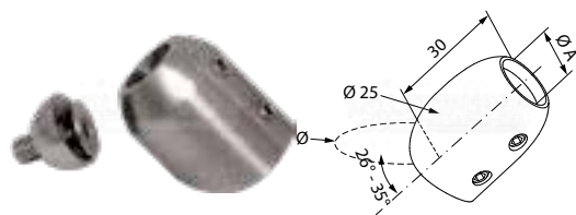
fissaggio per inclinazioni da 26^\circ a 35^\circ
