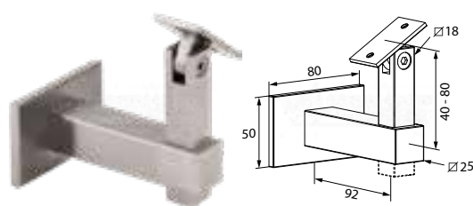
sostegno snodabile e regolabile con piastra
