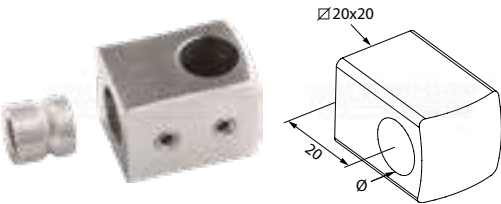
fissaggio con foro passante
